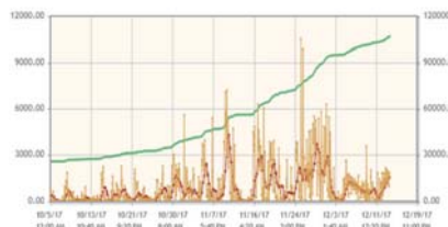
■ 24小时铁磁颗粒浓度 ■ 铁磁颗粒累计质量 ■ 1小时铁磁颗粒浓度
