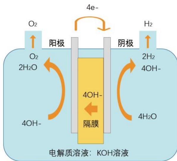
碱性水电解工作原理示意图
