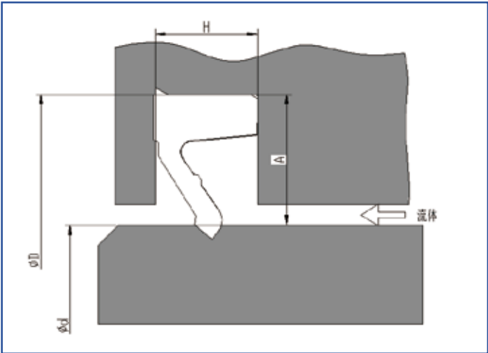
安装示意图 Installation diagram
