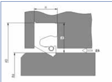
安装示意图 Installation diagram
