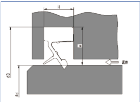
安装示意图 Installation diagram
