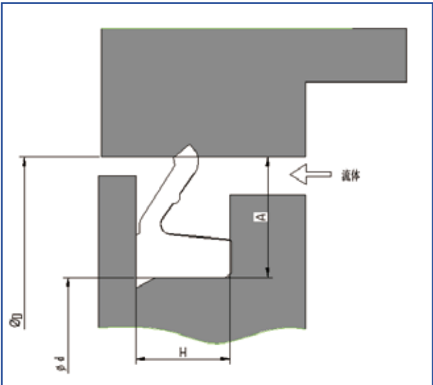
安装示意图 Installation diagram
