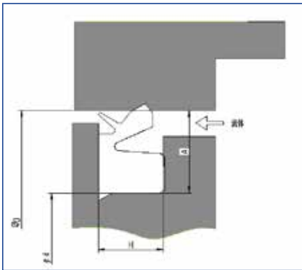
安装示意图 Installation diagram
